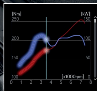
Courbes de puissance et de couple.
